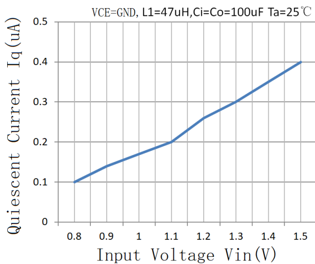
4、输入电压 VS. 静态电流
