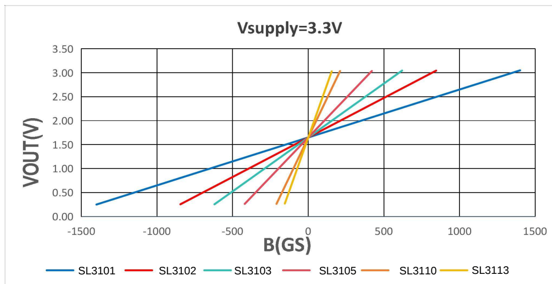
输出电压 VS 磁场 @VDD=3.3V
