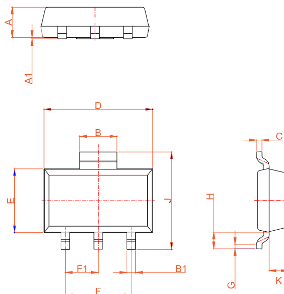
SOT-89
