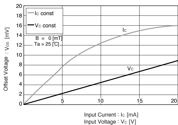
V os (V u )-V c , V os (V u )-I c
