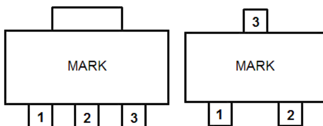
SOT89-3
